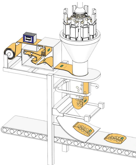
수직 충전 밀봉 포장기(VFFS)와 통합한 DataFlex®의 예
